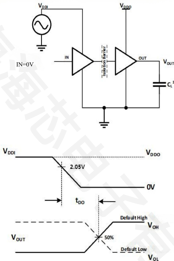
图 4. 默认输出延迟时间测试电路和电压波形
