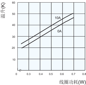
线圈温升
