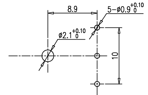
安装尺寸图
