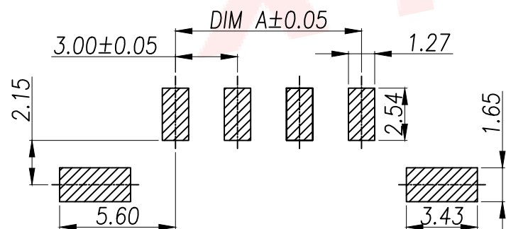
P.C.B Layout
