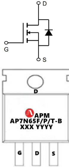
TO220-3L
