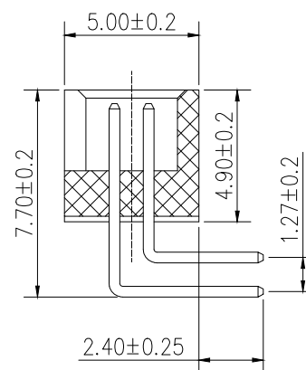
A-A SECTION
