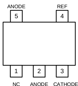
SOT23-5
