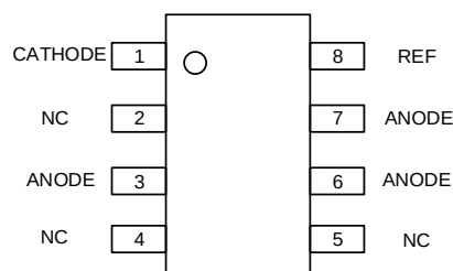
SOP8
