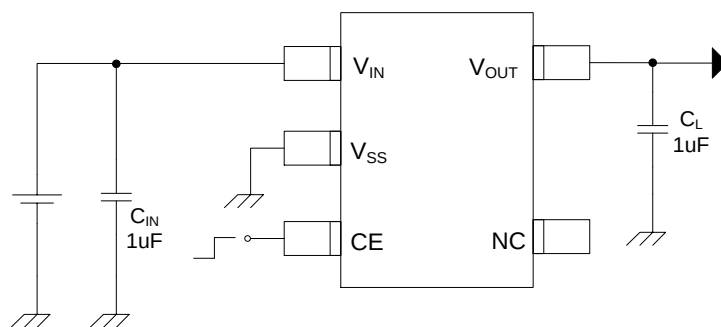
图 2. ME6211C 系列
