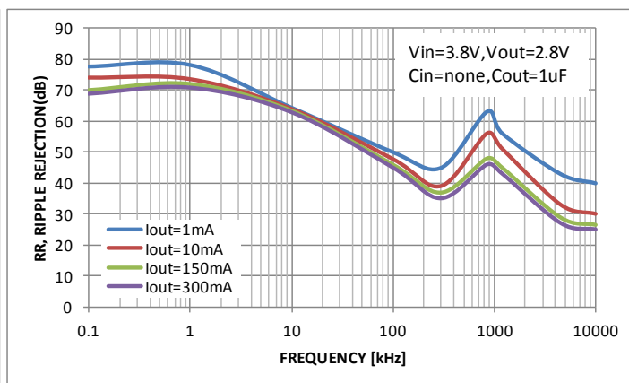
ME6211C28M5G
