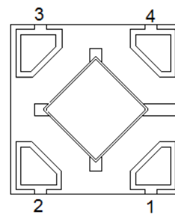
FBP1*1-4
