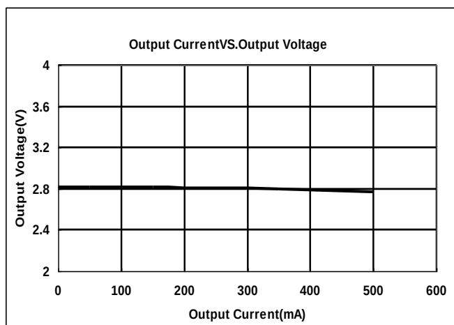
ME6211C28M5G
