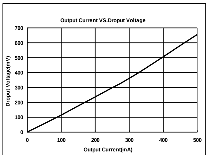
ME6211C28M5G
