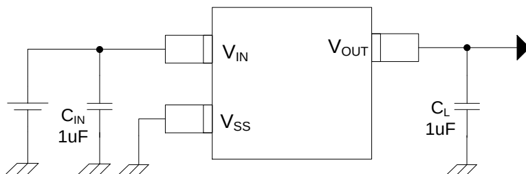
图 1. ME6211A 系列
