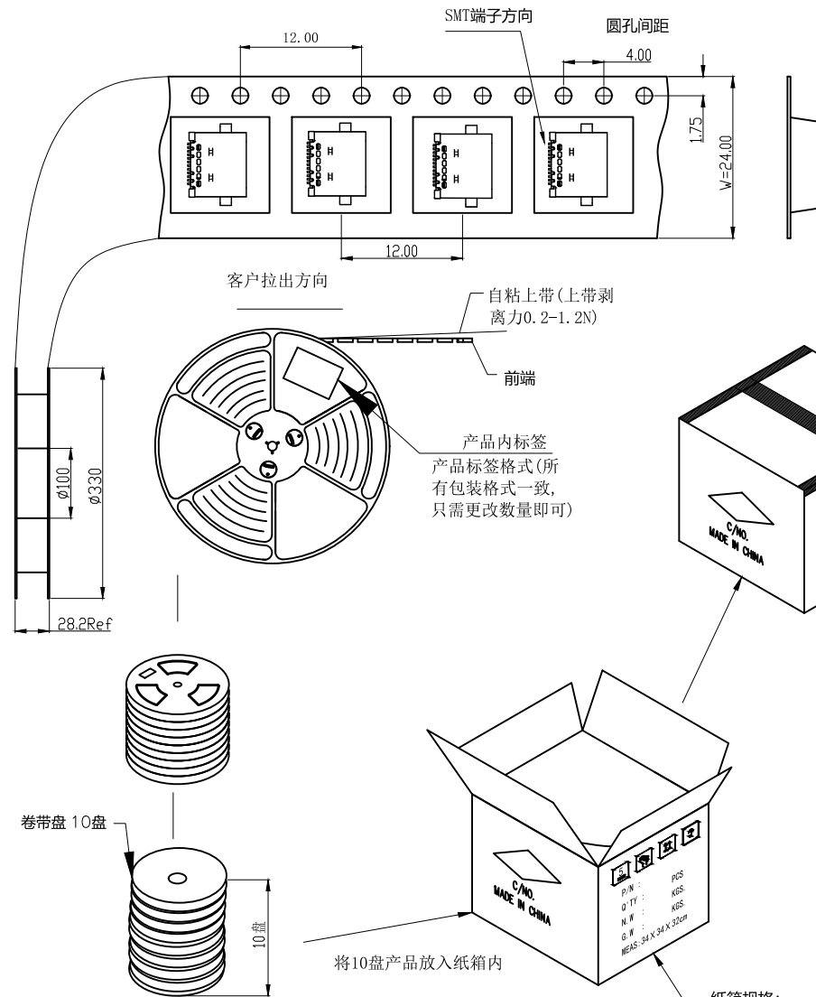
包装示意图:
