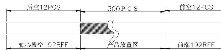
包装示意图:
