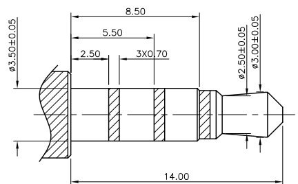
(&lt;math&gt;\phi 3.50\text{mm}&lt;/math&gt; 3 OR 4 POLE PLUG DETAIL DRAWING)
