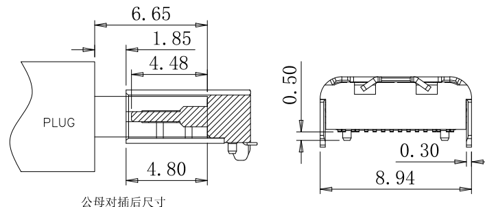
公母对插后尺寸
