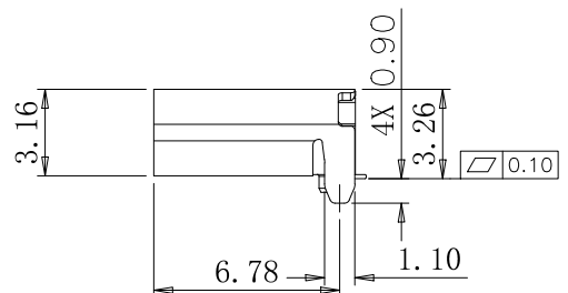
公母对插后尺寸
