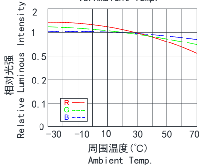
Fig. 3-相对光强与周围温度图 Relative Luminous Intensity vs. Ambient Temp.
