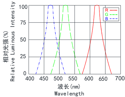
Fig. 1-光谱曲线 Spectrum Distribution
