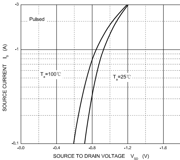
I_S — V_{SD}
