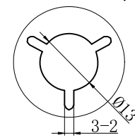
DETAIL: A 10:1
