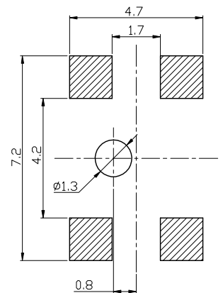
安装位置图
