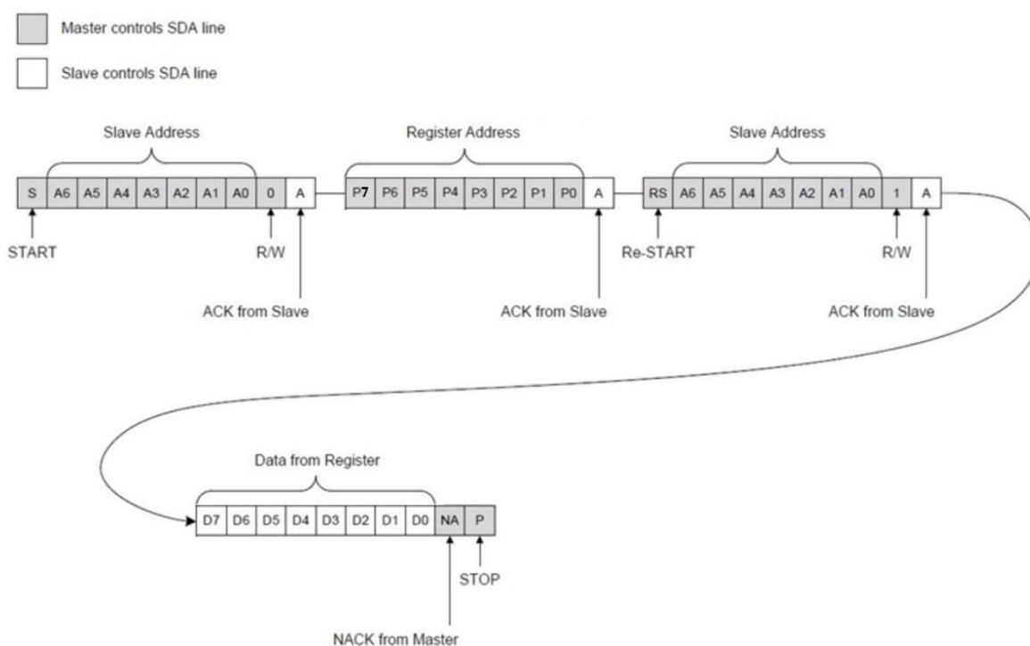
图 11.2-1 I 2 C 读时序
