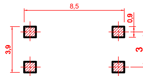
PCB. 焊接图
