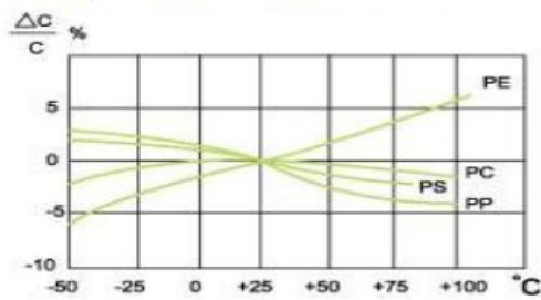
容量变化率与温度的关系
