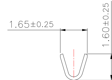
SEC:A-A
