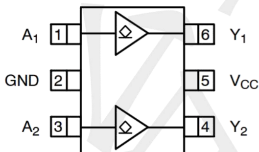
SOT363
