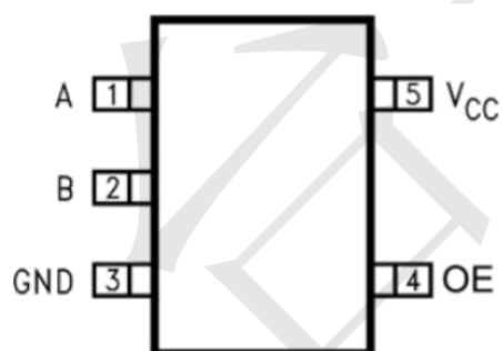
SOT23-5
