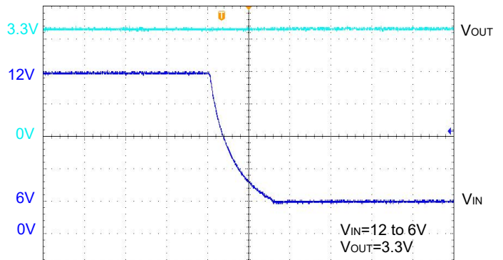
Input jump
