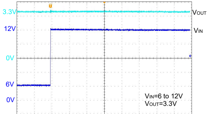
Input jump
