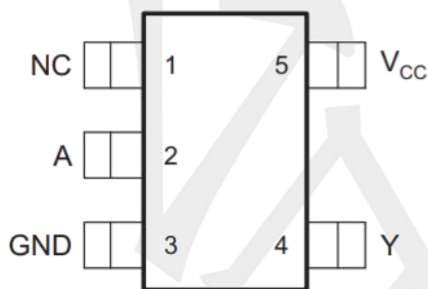
SOT353
