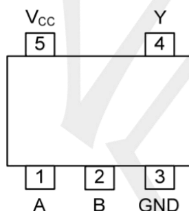
SOT23-5
