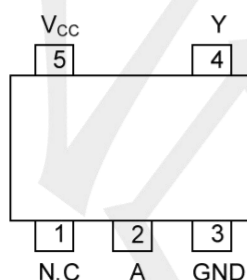
SOT23-5
