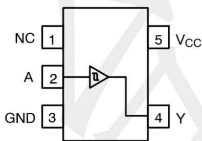
SOT353
