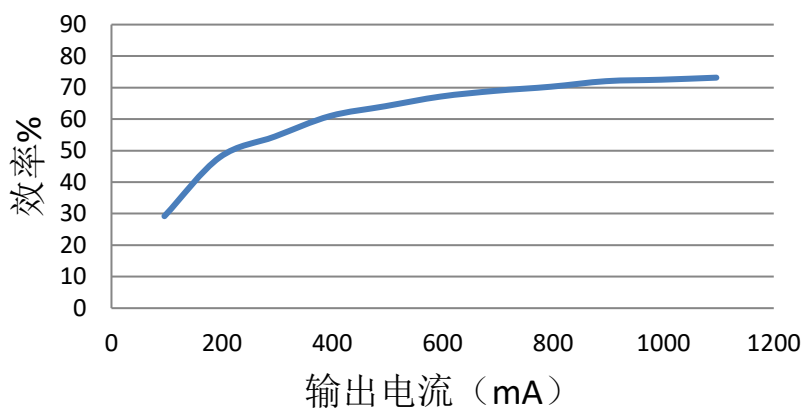
线圈2输入9V-10W效率曲线
