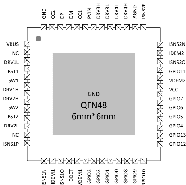
图 2 IP6862B 引脚图
