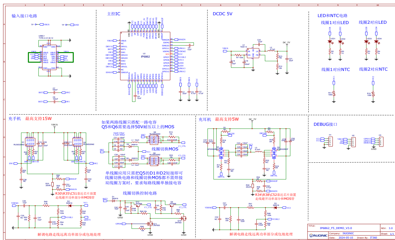
图 21 典型应用原理图
