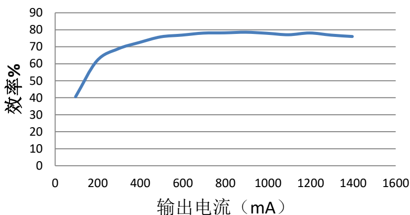
线圈1输入5V-5W效率曲线
