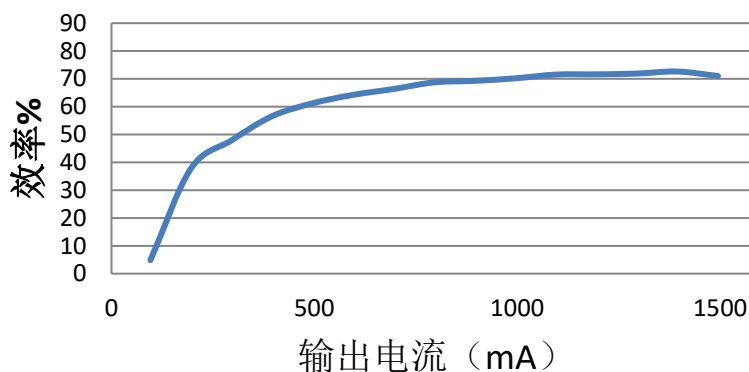
线圈2输入12V-15W效率曲线
