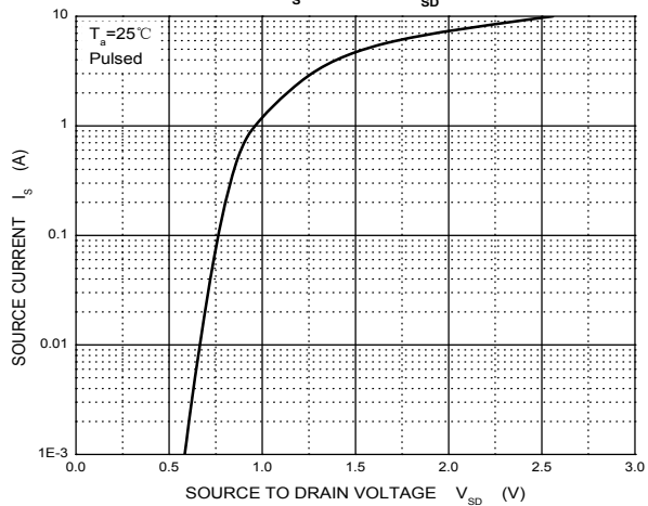
I_S — V_{SD}
