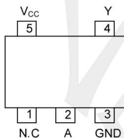
SOT23-5
