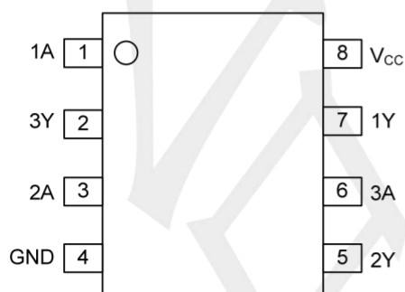
VSSOP-8
