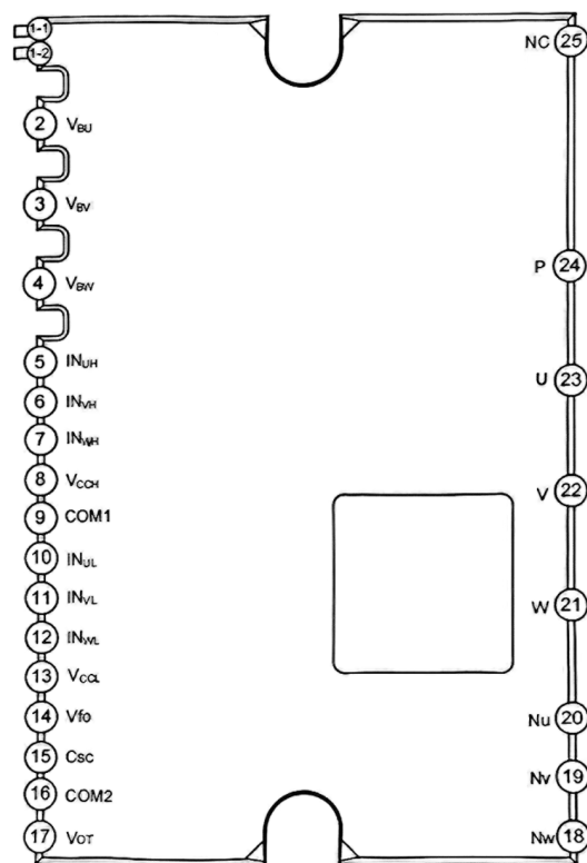
图 2：引脚定义图
