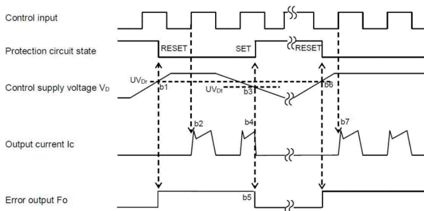
图 7：欠压保护（低侧）
