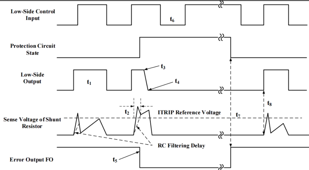
图 6：短路电流保护（仅针对下桥臂 / 低侧）
