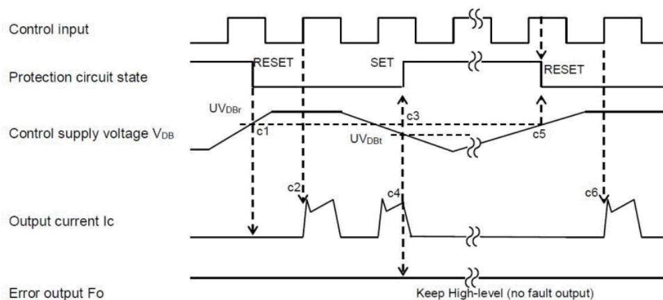
图 8: 欠压保护 (高侧)
