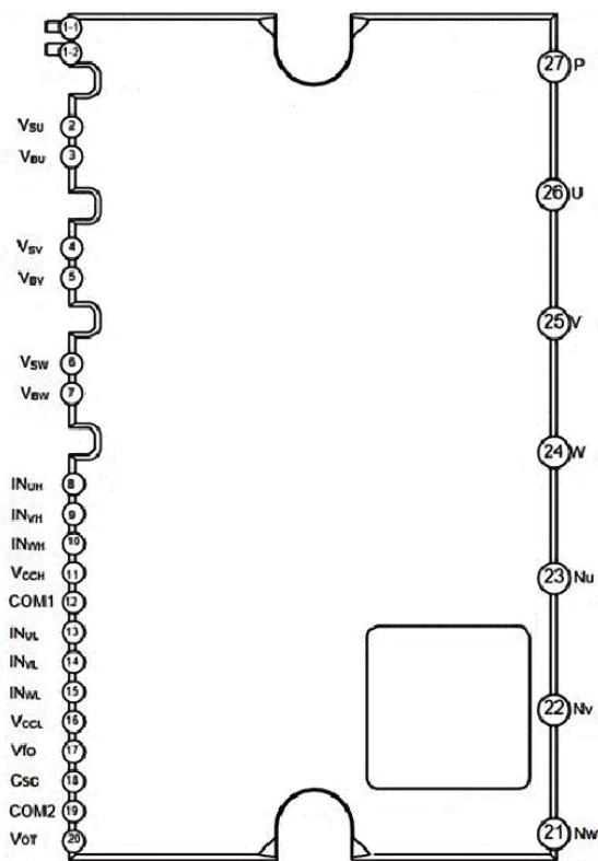
图 2：引脚定义图
