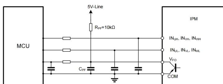
图 10：MCU 输入 / 输出连接电路（推荐方案）
