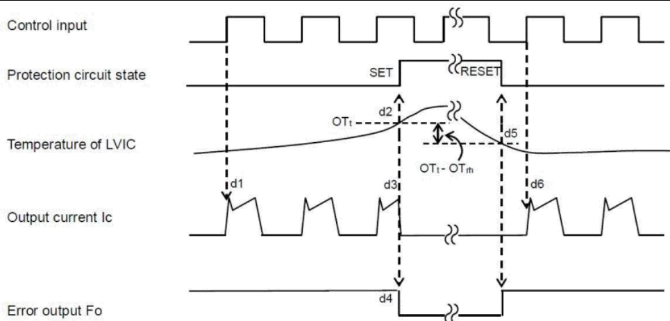
图 9：过温保护（仅低侧）
