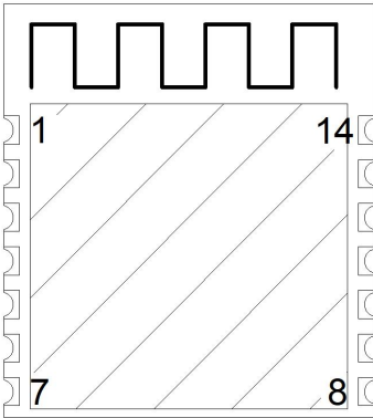
图 2.2：HJ-01B 引脚分布图（正面图）
