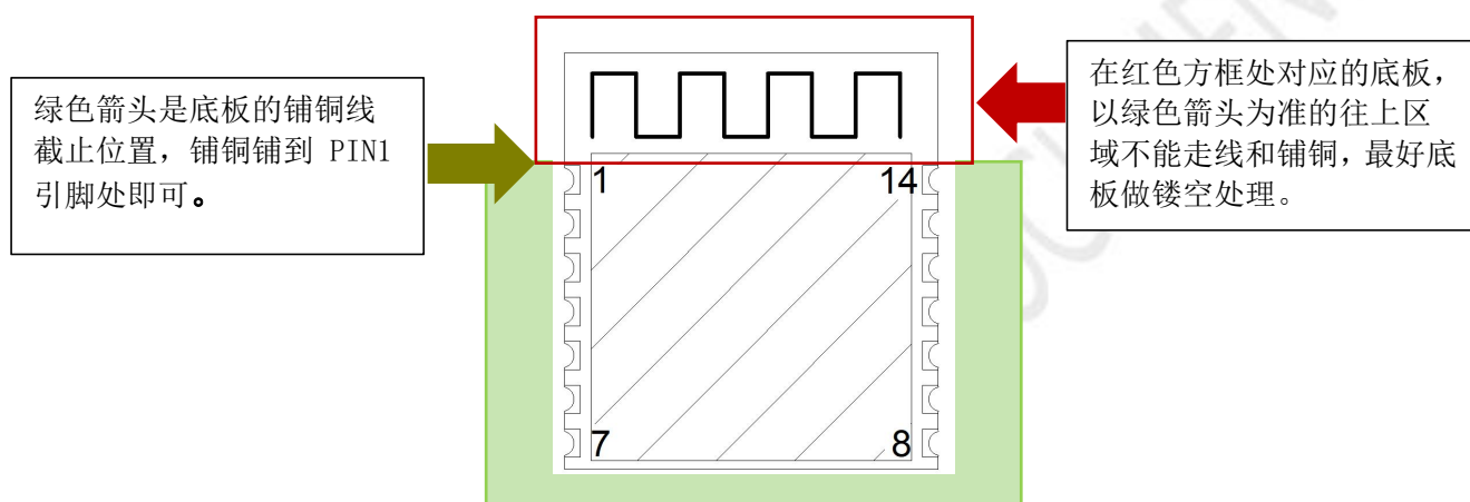
图 3.1：模组放置建议
