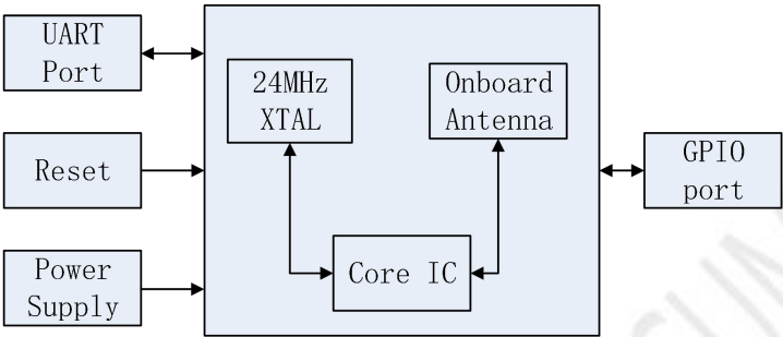
图 2.1：HJ-01B 功能框图
