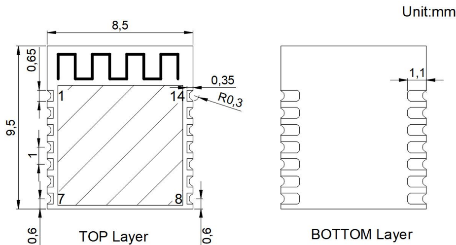
图 6. 1：HJ-01B 机械尺寸图
