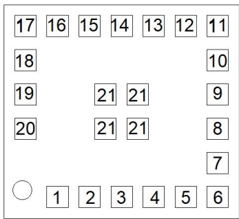
图 2.2：HJ-180IMH-15 引脚分布图（正面图）
