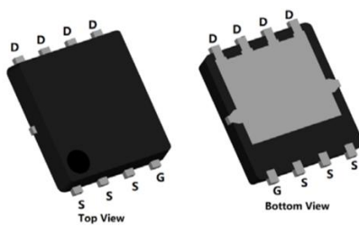
PDFN5X6-8L
