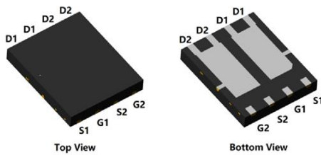
PDFN5X6-8L
