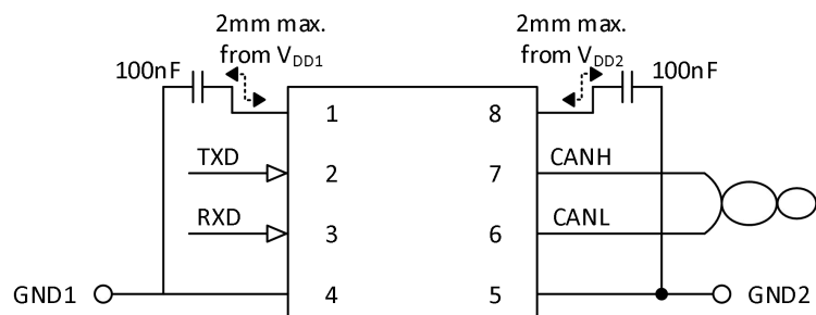
Fig. 6. 典型参考设计示意图
