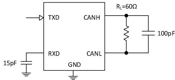
Fig. 4. 收发器时序测试电路图
