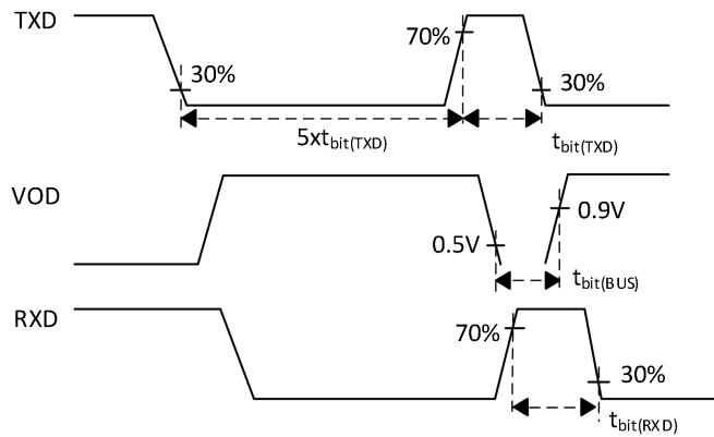
Fig. 2. t_{\text{bit}} 延时示意图
