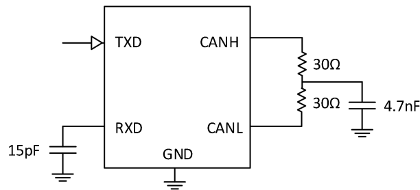
Fig. 5. 收发器总线对称测试电路图
