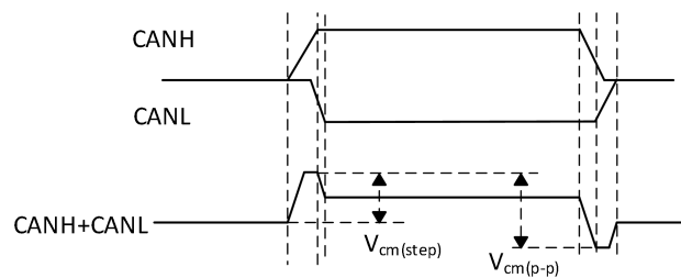
Fig. 3. 总线共模电压
