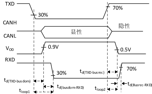
Fig. 1. 收发器传输延时示意
