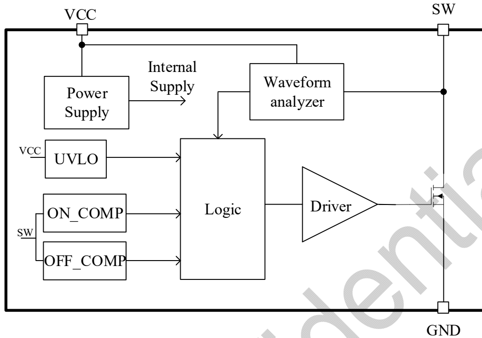
图 3. S7303S 内部框图
