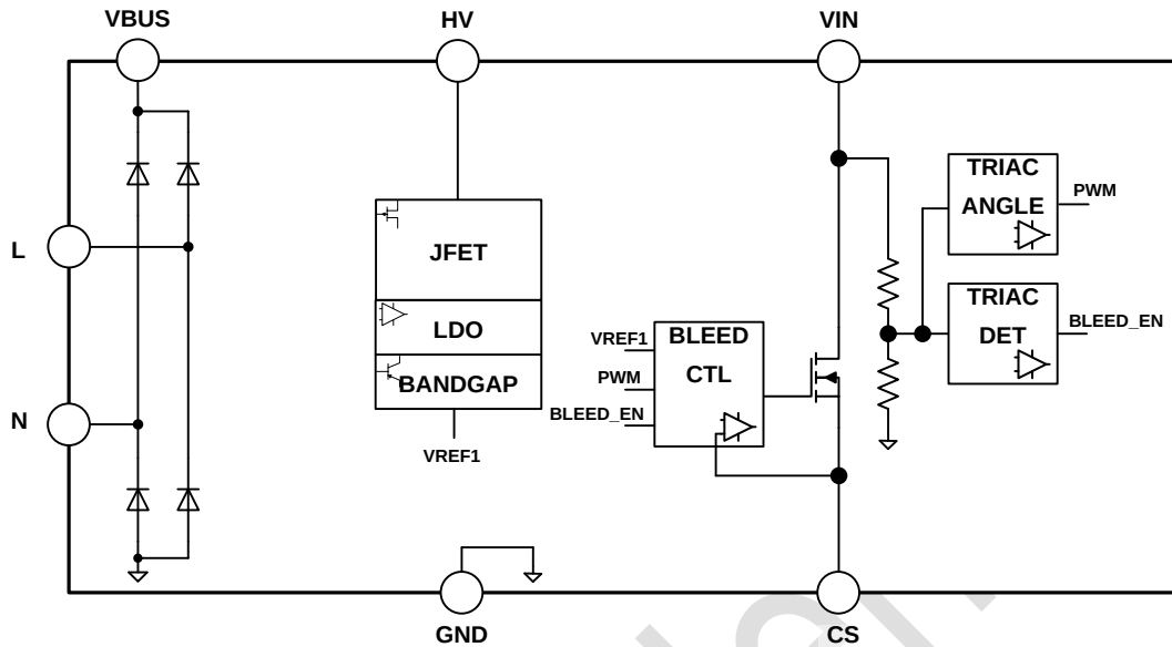
图 3 BP5177GB 内部框图
