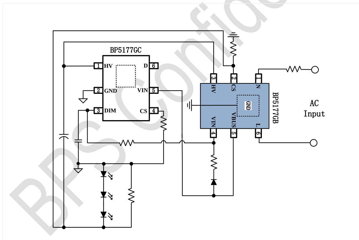
图 1 BP5177GB 典型应用图
