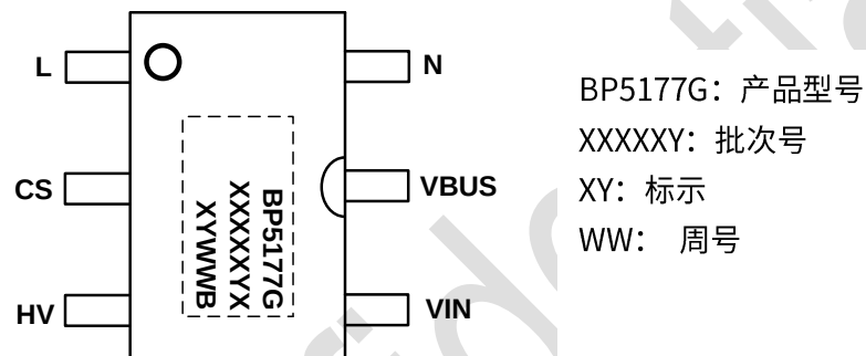
图 2 管脚封装图
