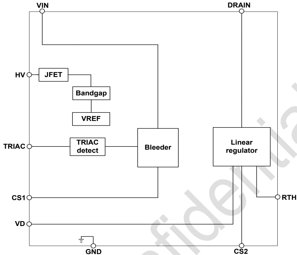
图 3 BP5188GSN 内部框图
