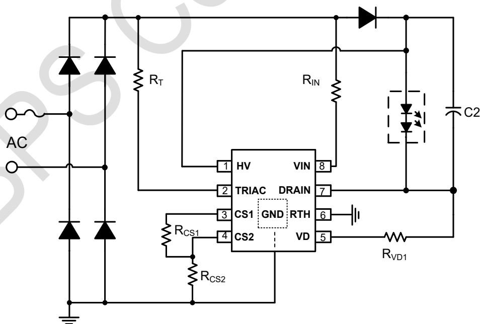
图 1 BP5188GSN 典型应用图
