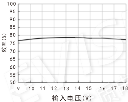
效率Vs输入电压(满载) WRB1205S-3WR2
