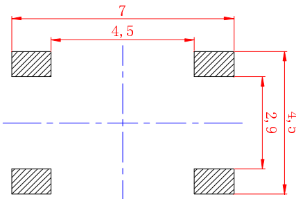
P C B 参考图
