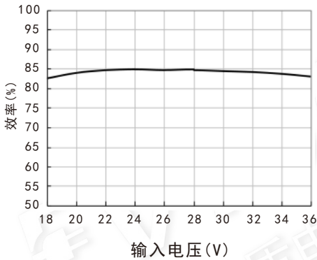
效率Vs输入电压(满载) WRE2415S-3WR2
