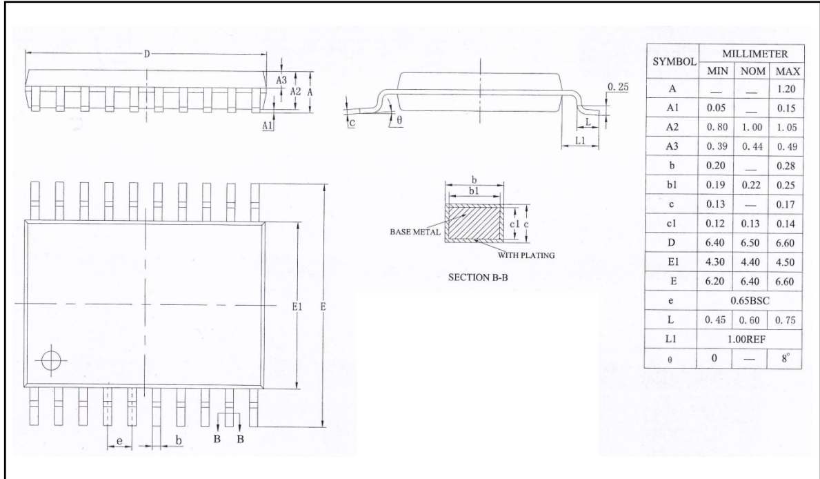
FIGURE 16 : TSSOP20 Package dimensions
