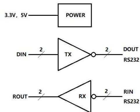
图2: HG3232A 逻辑图
