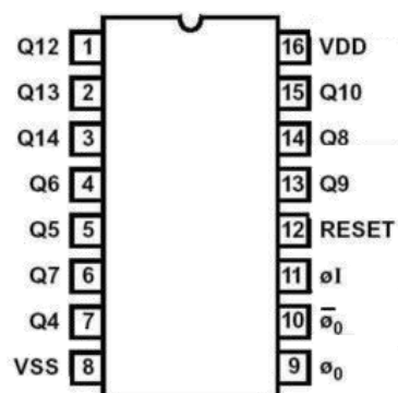
DIP-16/SOP-16/TSSOP-16
