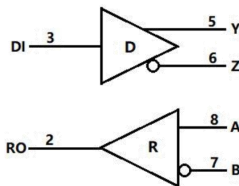
图 2：MAX490E 逻辑图
