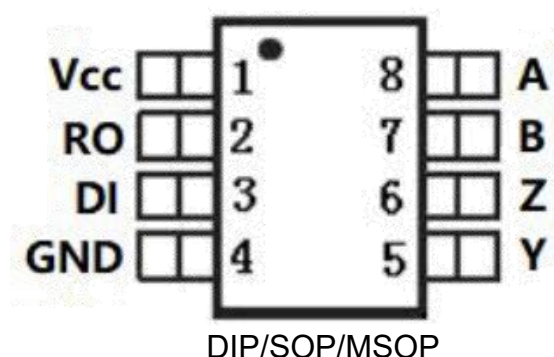
图 1：MAX490E 引脚图
