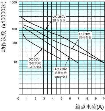
电耐久性曲线图 (2Z)
