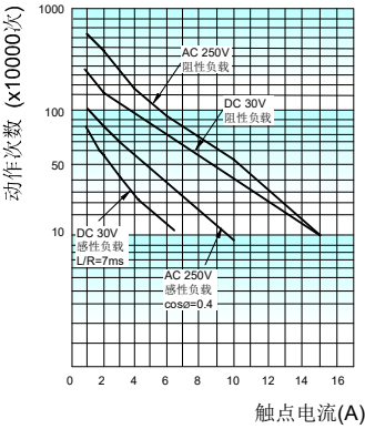
电耐久性曲线图 (1Z)
