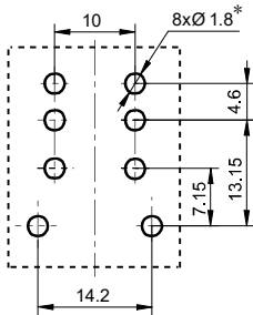
安装孔尺寸 (底视图)
