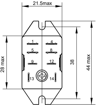
外形图
