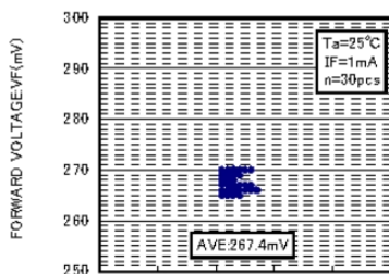
VF DISPERSION MAP
